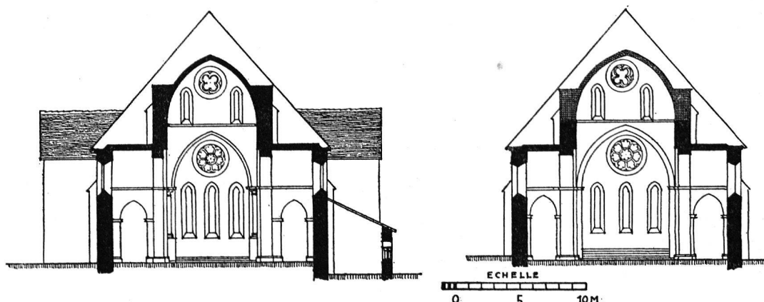
Fig. 7. Coupes transversales des églises abbatiales de Hauterive (à gauche) et de la Maigne (à droite), vers 1200
