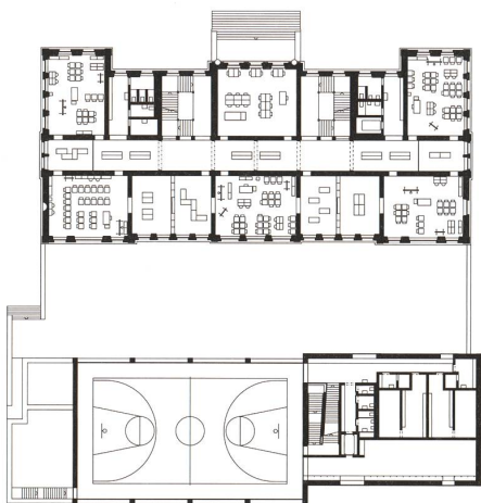
1. Obergeschoss
