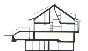
Querschnitt «Flarz 1»
