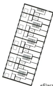
1. Obergeschoss
