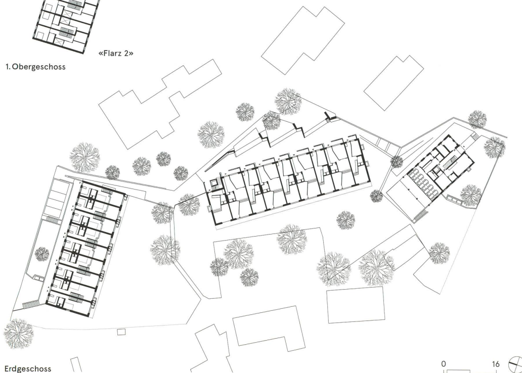
Erdgeschoss
