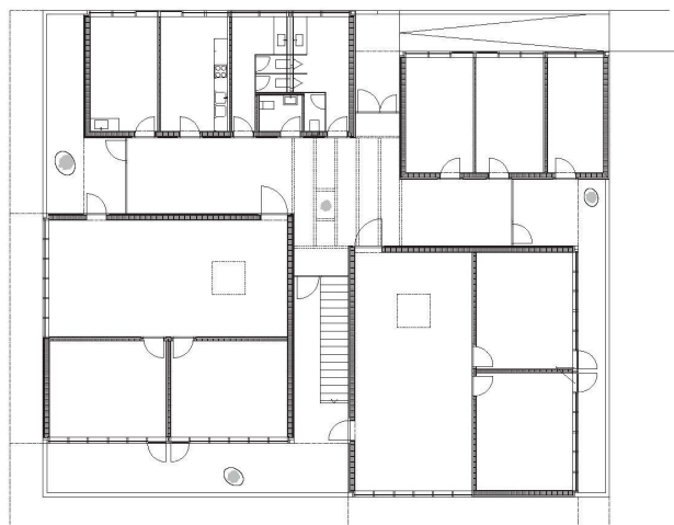
Hauptgeschoss
