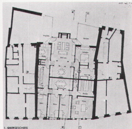
1. OBERGESCHOSS
