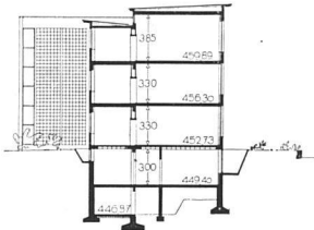
Querschnitt Klassentrakt
