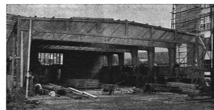
Abb. 6 Aufgerichtete Nagelbinder
