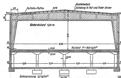
Abb. 7 Querschnitt 1:200 mit Fichte für 1,5 t pro m 2 Nutzlast über Kellergeschoß und genagelte Rahmenbinder über Erdgeschoß. Spannweite ca. 17 m, Binderabstand 4,2 m
