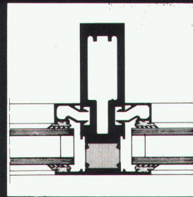
Bankgebäude der Schweizerischen Kreditanstalt in Wetzikon/ZH. Aluminium-Fassade mit vollisolierten Fenstern, Modell Alsecc-50.
