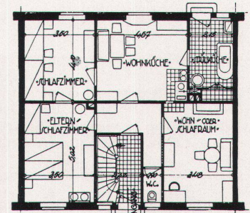
8 Grundriss einer 4-Zimmer-Wohnung
