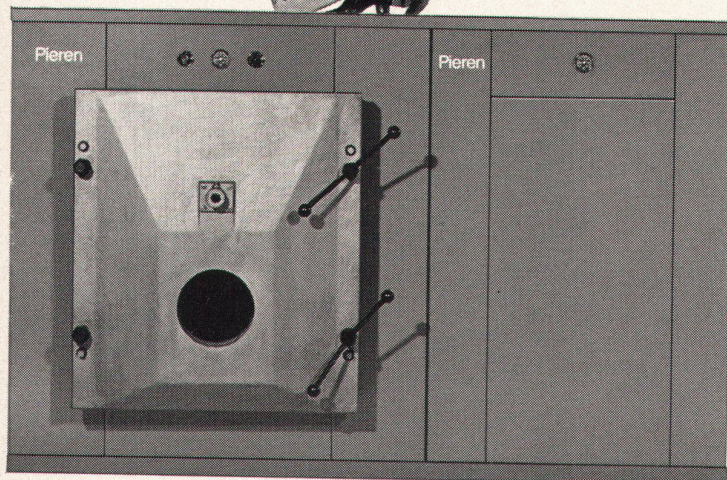
meteor SL Strahlungs-Heizkessel mit Batterieboiler
