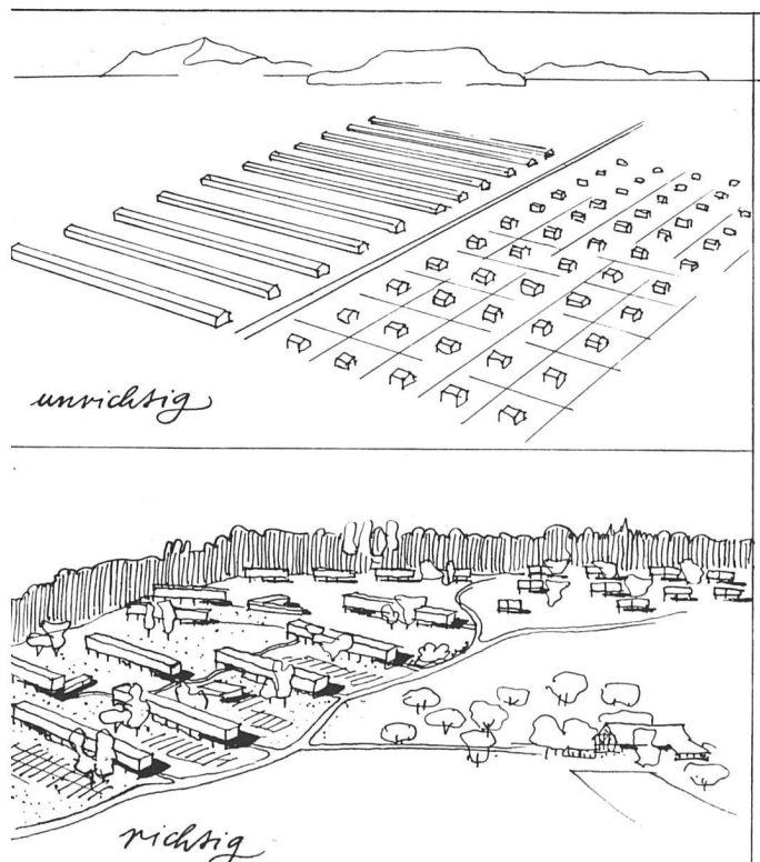
1bb. 1 Oben: Barackenstadt und schematische Einzelhaussiedlung in öder Gegend. Unten: Aufglockerte Notsiedlung in ansprechender Landschaft
