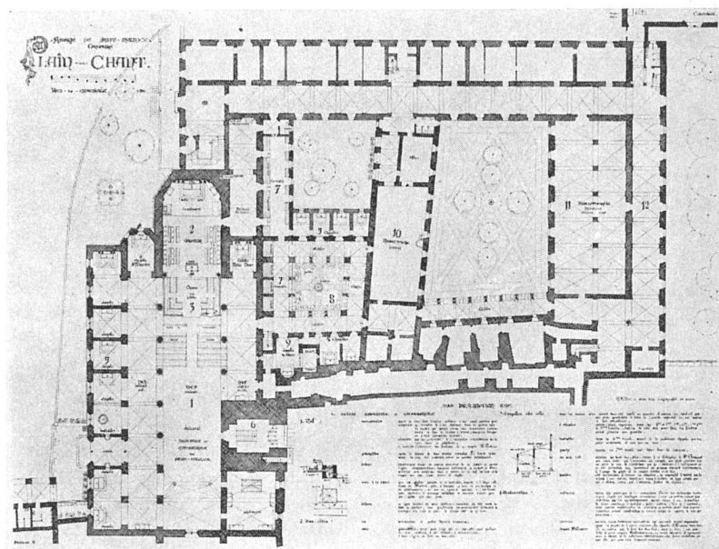
Erstprämiertes Wettbewerbsprojekt für die Erweiterung der Abtei St. Maurice, von Claude Jaccottet, Architekt, Lausanne. Grundriß 1:1000
