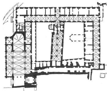
Grundriß des gegenwärtigen Zustandes
