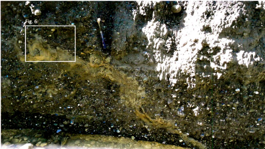
Fig. 5: Der Dyke im Frühling 2016. Man beachte, dass er sein Umgebungslockergestein (basale kiesige Lage mit überlagernder dünner Siltschicht) ohne merkliche Störung diskret durchschlägt, und dass er sich nicht mit seiner Umgebung zu vermischen scheint.
