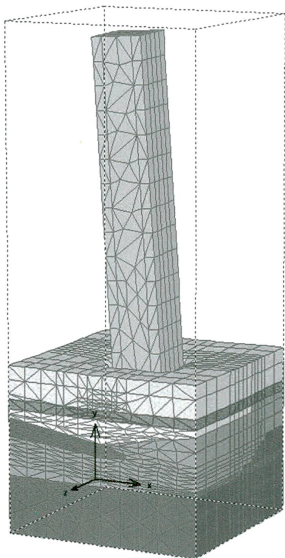
Fig. 5: Città di Castello tower mesh for the FEM analysis.
