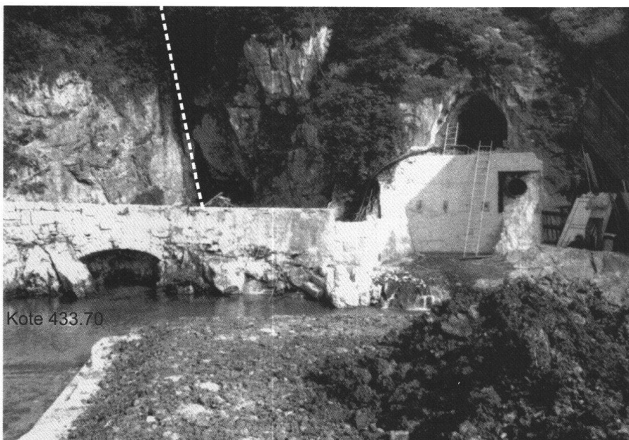
Fig. 3: Quellteich der Brunnmühlequelle mit der subvertikalen, NNW-SSE streichenden Quellklüfte (gestrichelte Linie) in den Oberen Twannbachkalken. Rechts erkennbar der heute zugemauerte Zugangsstollen zum Ligerztunnel.
