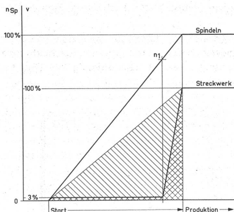
Abb. 7 Hochlaufprogramm
