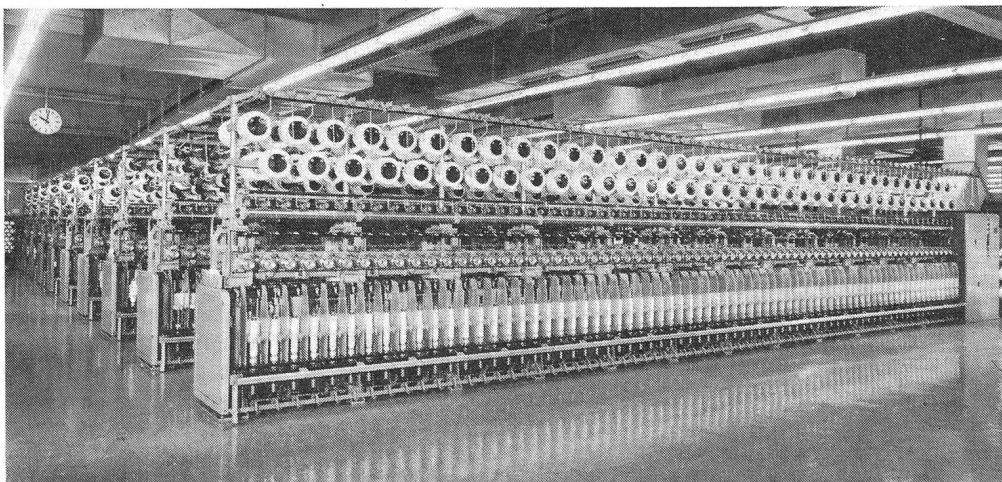
Abb. 1 Rieter-Streckzwirnmachine Typ J5/10
