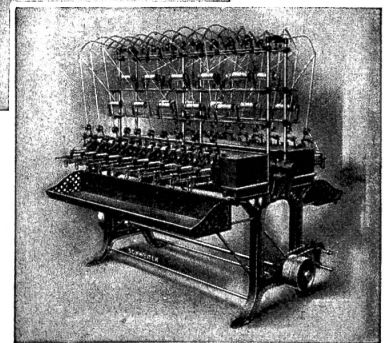
Kreuzschuß-Spulinmaschine Typ BUA. „Klein-Rapid“
