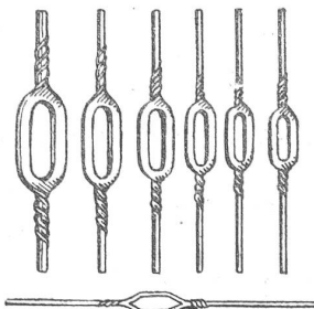
Universallitzen mit eingesetztem Stahlring
