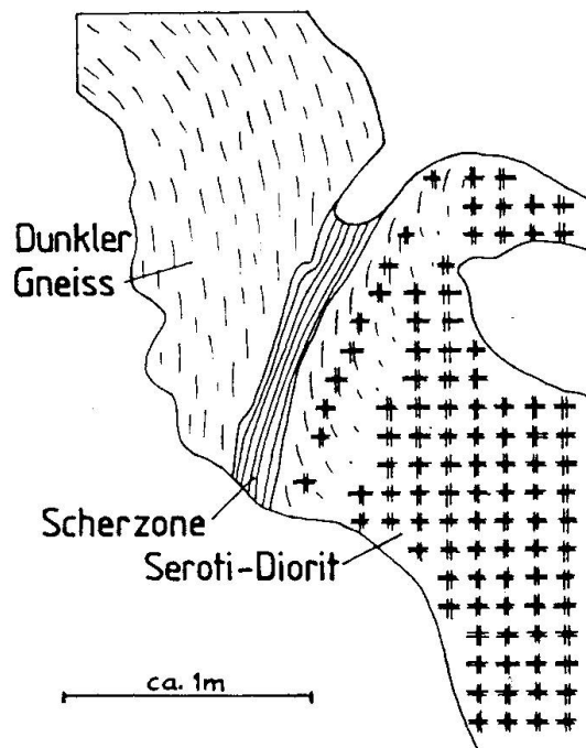
Abb. 2 Ein typischer Kontakt des Seroti-Diorits zu seinem Nebengestein: Eine zum Kontakt parallele Scherzone, in die die Schieferung des Dunklen Gneisses einbiegt, die in einigen m Entfernung eine deutlich andere Richtung hat. Der Übergang von der Scherzone zum massigen Seroti-Diorit ist ebenfalls ein allmählicher. (Schematische Zeichnung nach einem Foto. Km-Koord.: 2657N/0507E)
