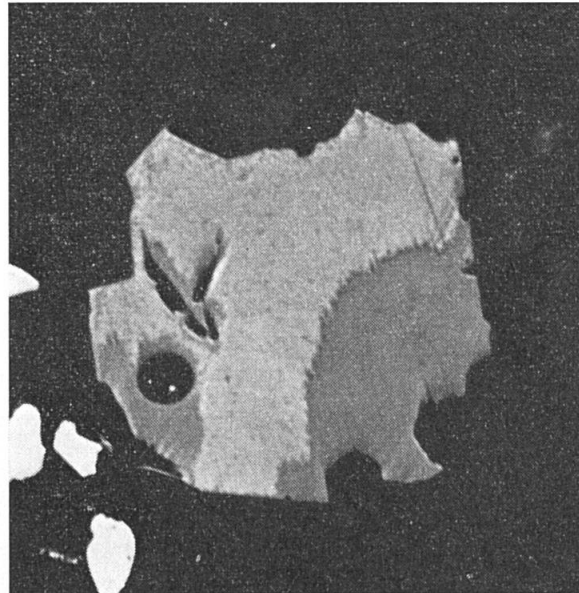
Fig. 5. Katzenbuckel/Odenwald. Natronshonkinit. Xenomorpher Pseudobrookit mit heller, reflektierender Polier- und Oxydationshaut. Daneben Eisenglanz-körnchen: weiss. Verg. 1400mal (Nachvergrösserung einer 650mal-Aufnahme), Ölimmersion.
