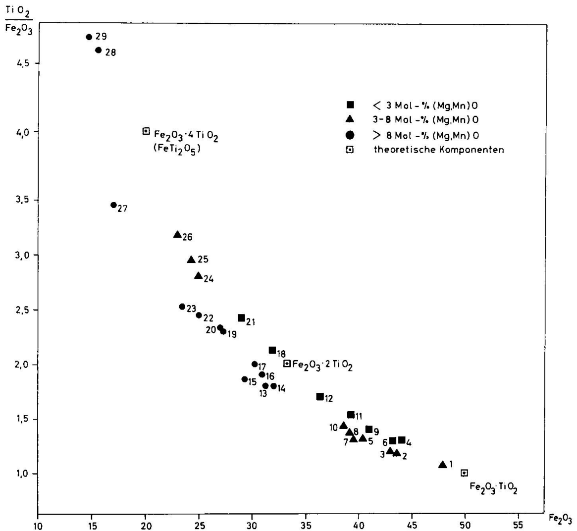
Darstellung der Pseudobrookit-Analysen Mol-Quotient \text{TiO}_2/\text{Fe}_2\text{O}_3 gegen Mol-% \text{Fe}_2\text{O}_3
