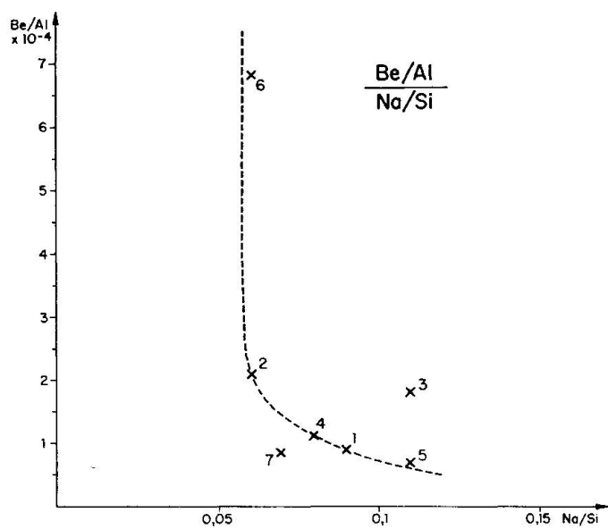
Fig. 13. Diagramm Be/Al Na/Si.
