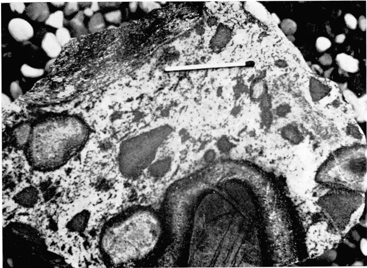
Fig. 7. Sphärolithische Breccie mit Zonen von Olivin-Talk-Pennin-Klinochlor-Hornblende-Biotit. Vadrec da la Trubinasca, 2200 m.
