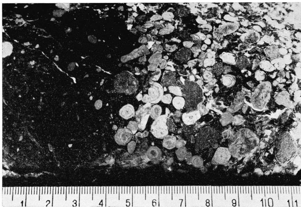
Fig. 1. Bohrkern aus Böhnerz, Limberg, ca. 2663. m. Rechts = unten. Dunkel = roter Bolus, hell = ockerfarbene Bohnen aus Kaolinit + Goethit. Grau, meist körnig aussehend = Hämatit. Weiss = schlierige Adern aus fast reinem Kaolinit.
