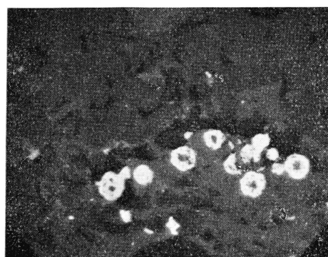
Fig. 6. Pechblende mit Andeutung von Idiomorphie. 200 \times .
