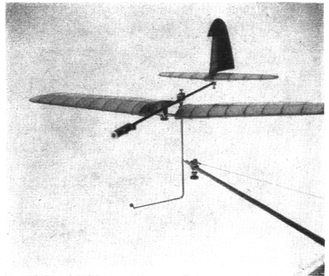
Fig. 21 Das Seitenruder hat gegenüber der Seitenstabilitätsfläche einen Anstellwinkel erhalten. Entsprechend demselben ändert der Rumpfstab seine Richtung
