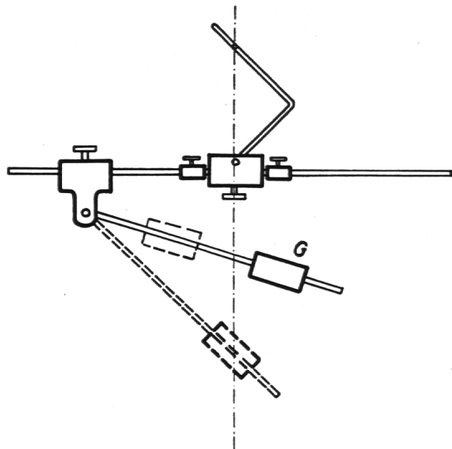
Fig. 18 Mittelt Stab mit Bride kann der Schwerpunkt vor- oder rückwärts, hoch oder tief genommen werden
