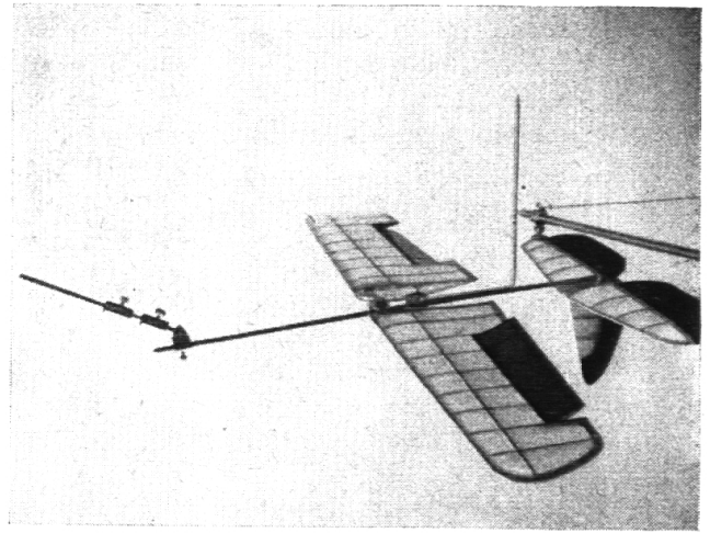
Fig. 24 Das Modell hat sich mit Hilfe der Querruder in die Rückenlage gedreht und bewegt sich nun in die Ausgangslage zurück, um die Rotation von neuem zu beginnen
