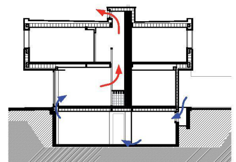
05 Schema natürliche Belüftung (Pläne: Christian von Düring)
