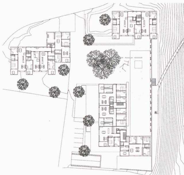
Links der Neubau, rechts die beiden noch bestehenden Gebäude, die umgebaut werden. Das südliche Haus wird zusätzlich mit einer Wohnung erweitert (Weiterbearbeitung, Staufers & Hasler)
