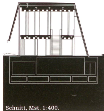
Schnitt, Mst. 1:400.
