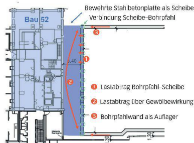
Oben: Situation Baugrube mit Nachbargebäuden aus den 1950er- und 1960er-Jahren. Unten links: Baugrubenschnitt auf der Westseite bei Bau 52. Unten rechts: Tragverhalten.
