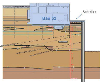
Oben: Situation Baugrube mit Nachbargebäuden aus den 1950er- und 1960er-Jahren. Unten links: Baugrubenschnitt auf der Westseite bei Bau 52. Unten rechts: Tragverhalten.
