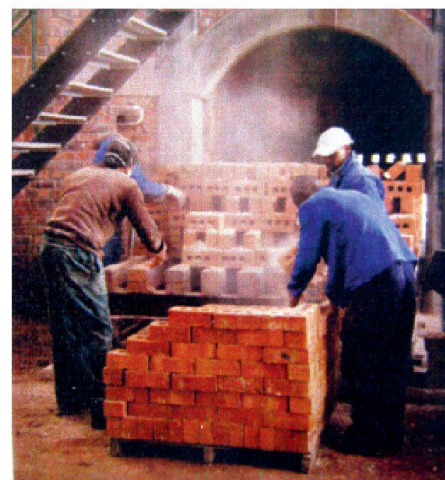
02 Arbeiter entnehmen die fertigen Ziegel (Bilder: VSBK-Projekt Südafrika)
