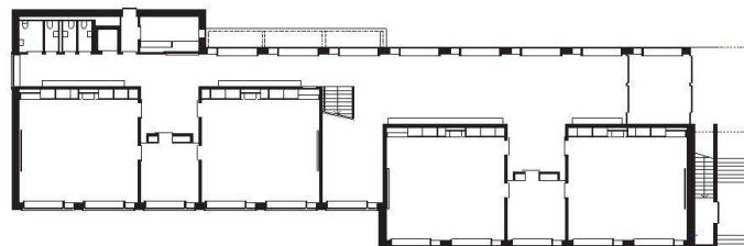
02 Grundriss Erdgeschoss, Mst. 1:600 (Pläne: Team 4 Architekten)
