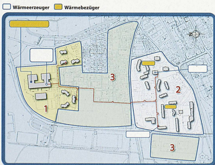
Wärmeverbundnetz Engerfeld in Rheinfelden. Links das Schulhaus Engerfeld, wo die neue Holzschnitzelfeuerung installiert wird. Sie wird mit den bestehenden Ölheizzentralen rechts im Bild verbunden (Grafiken und Bilder: Eicher + Pauli)
