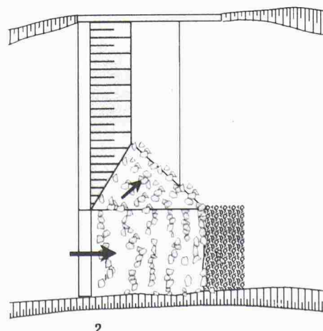
Anordnung von Fischrampen an Wehren (Pfeile: Fließrichtung über die Fischrampe). Beispiel siehe Bild 3 (Bild: Frank Krüger)
