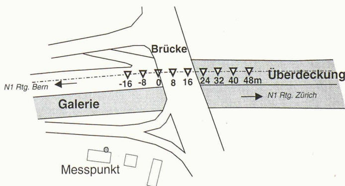
Die Lärm-Quellenpunkte und ein Messpunkt im Modellschema des Tunnel-Westportals
