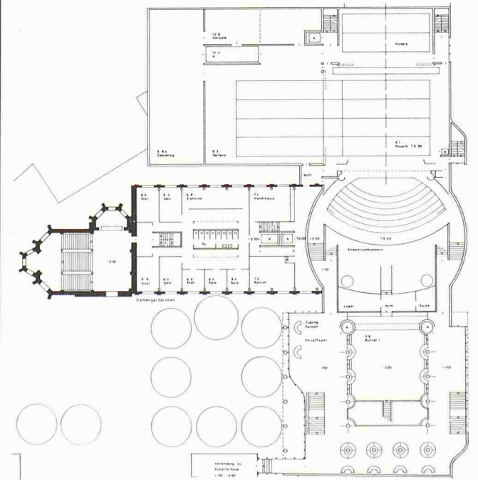
Parkett-/Bühnengeschoss
