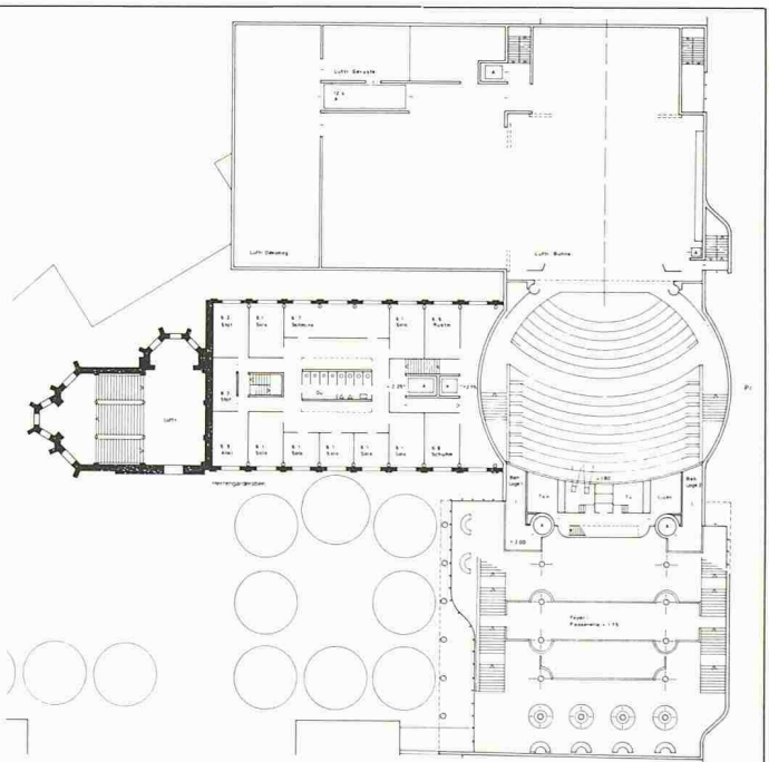
Parkett-, Bühnengeschoss
