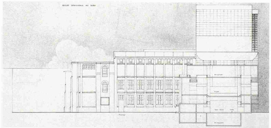
Ansicht Amerikahaus
