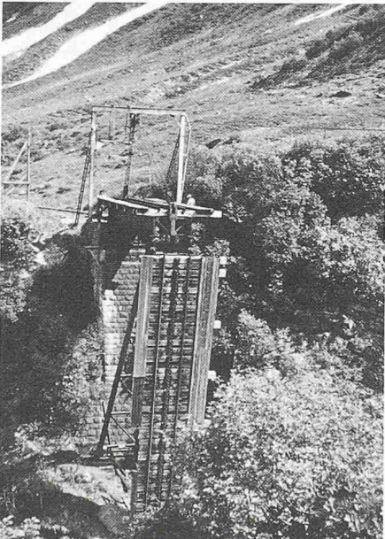
Steffenbachbrücke: Das talseitige Segment mit dem abgeklappten Mittelteil ist ausgezogen und kann auf das Widerlager abgesehen werden
