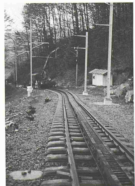
Bild 2. Provisorisch montiertes Zahnstangengleis
