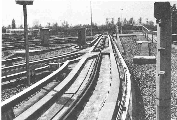
Bild 4. Betriebshof beim Endpunkt «Quatre Cantons». Deutlich sind die Tragbalken und die Seitenführungen erkennbar. Wo letztere unterbrochen werden müssen, übernimmt eine mittlere Leitschiene mit Hilfe eines am Fahrzeug angebrachten Lenkzapfens die Seitenkontrolle. (Bild: Verfasser)
