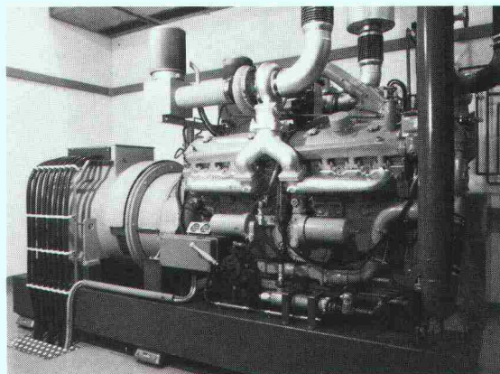
Notstromgruppe 500 kVA
