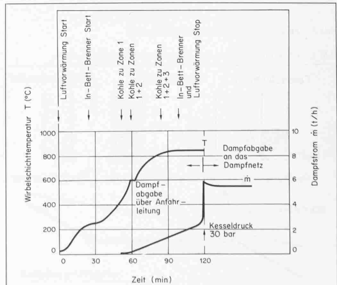
Bild 5. Anfahrtdiagramm
