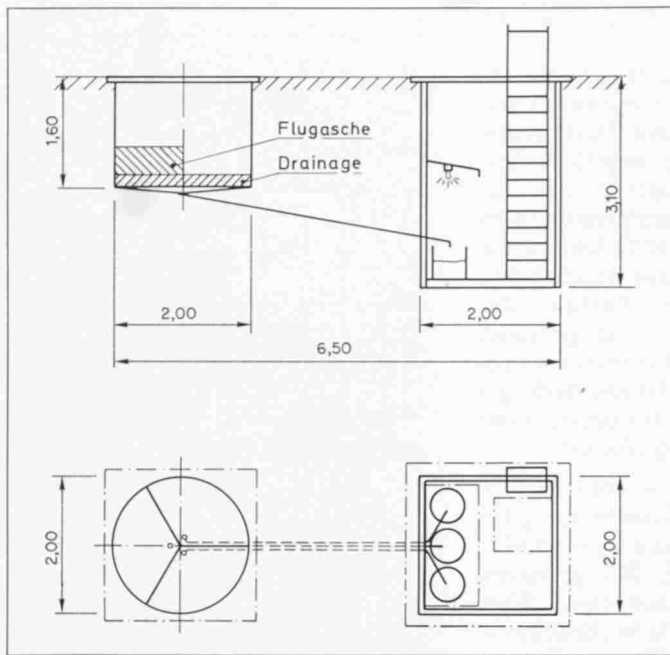
Bild 8. Granulierter Flugstaub aus dem Tuchfilter, in einem Deponiebehälter den natürlichen Wetterbedingungen ausgesetzt. Versuchsanordnung.
