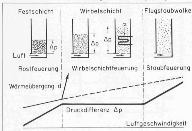
Bild 1. Charakteristika und Einordnung der Wirbelschichtfeuerung
