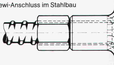
Gewi-Anschluss im Stahlbau
