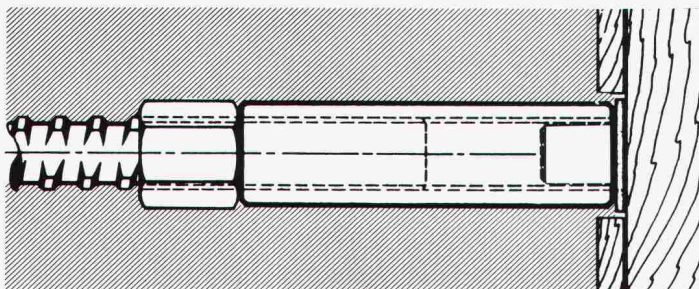
Gewi-Muffenstoss
