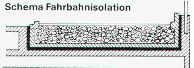
Schema Fahrbahnisolierung
