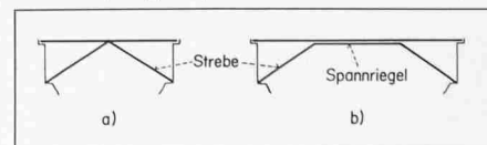
Bild 2. Sprengwerkformen
