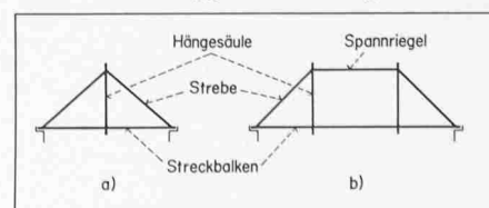
Bild 3. Ausbildungsformen von Hängewerken
