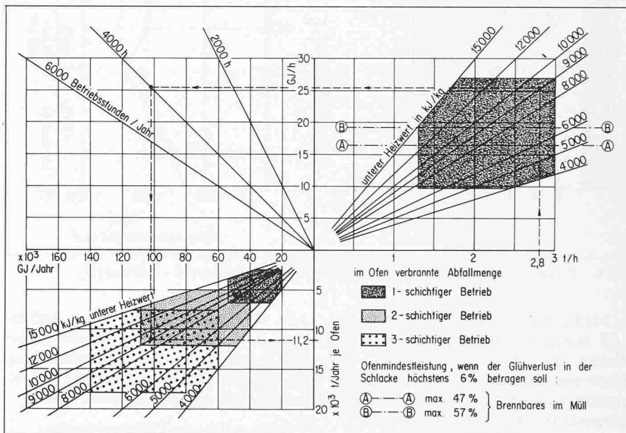
Bild 7. Feuerungsmomogramm für einen Müllofen für 3 t/h
