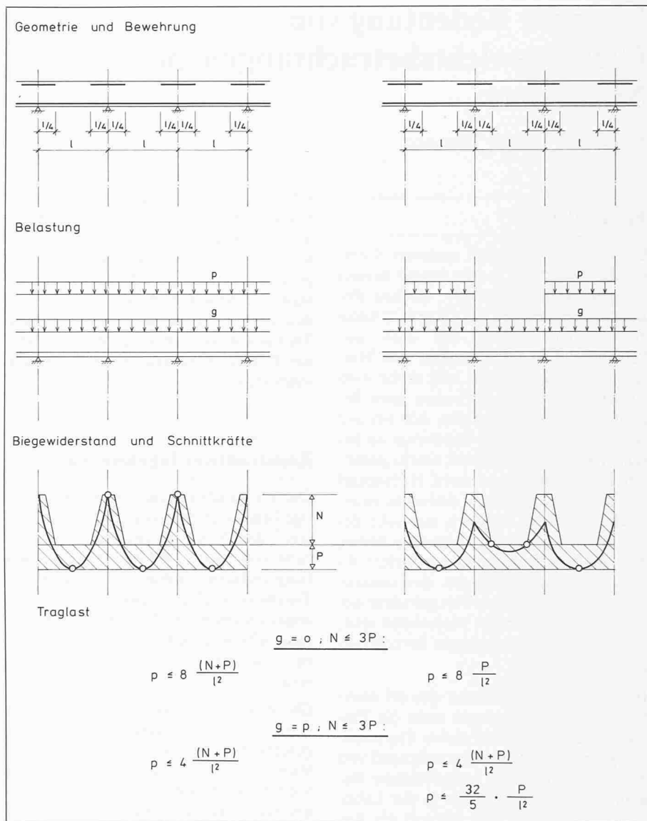
Bild 2. Durchlaufender Stahlbetonträger
