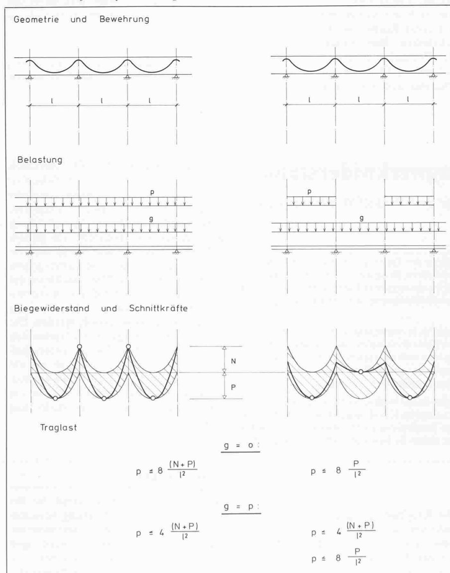
Bild 1. Durchlaufender Spannbetonträger
