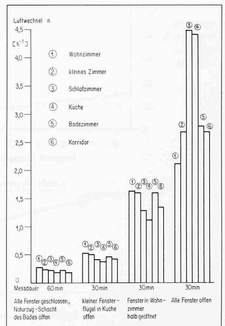
Bild 3. Messresultate für den Luftwechsel in den verschiedenen Räumen einer Wohnung ( t_{\text{ausser}} um -1 \text{ }^\circ\text{C} ; Windgeschwindigkeit etwa 6,5 \text{ m/s} )
