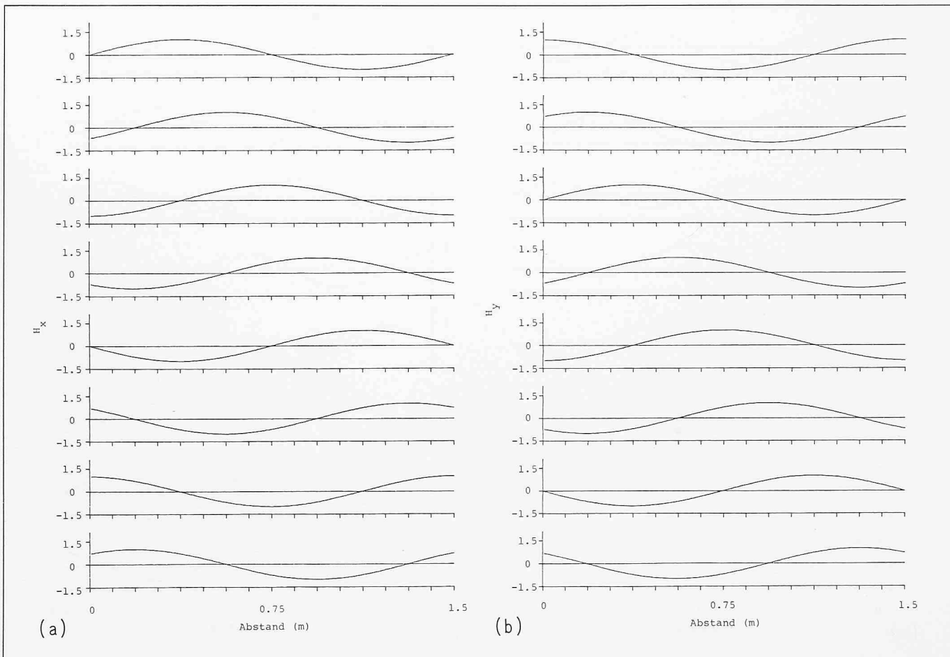
Bild 13. Feldkomponenten H_x und H_y , dargestellt als Funktion von x für acht verschiedene Zeiten innerhalb einer Periode (Gleichung IV.2 und IV.3 nomiert)
