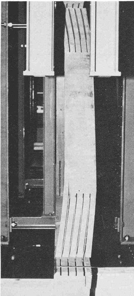
Bild 9. Knickfigur eines Druckstabes eines Fachwerkes mit biegeelastischem Anschlussbereich
