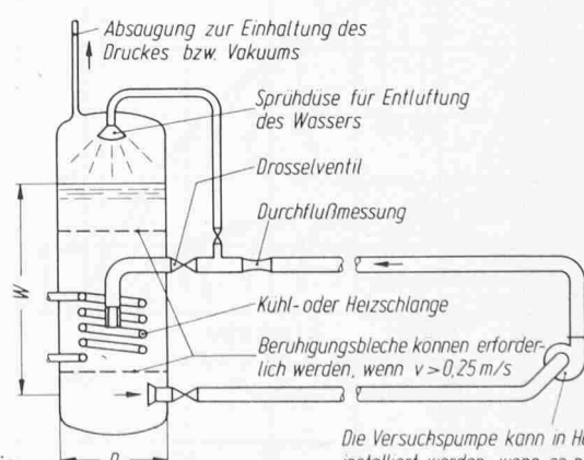
Bild 3. Kavitationsversuch. Änderung der \text{NPSH}_{\text{vorh}} in einem geschlossenen Kreislauf
