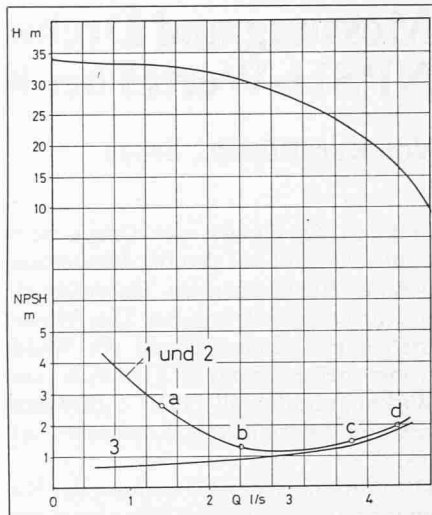
Bild 5. NPSH-Werte bei: 1 Änderung des Saugwasserspiegels 2 Drosselung saugseitig 3 Förderung in einem geschlossenen Kreislauf. Die eingezeichneten Punkte a-d entsprechen den Versuchswerten in Bild 4 und Tabelle 1
