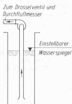
Bild 1. (links) Kavitationsversuch. Änderung der \text{NPSH}_{\text{vorh}} durch Änderung des eintrittsseitigen Flüssigkeitsspiegels
