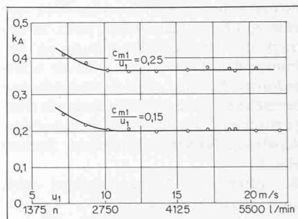
Bild 8. Abhängigkeit der Kavitationszahl k_A von der Drehzahl und der Umfangsgeschwindigkeit am Radeintritt. Versuche mit Wassertemperatur 49,5 °C K. Graumann [4]
