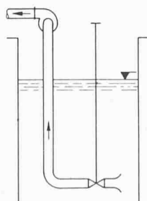
Bild 1. (links) Kavitationsversuch. Änderung der \text{NPSH}_{\text{vorh}} durch Änderung des eintrittsseitigen Flüssigkeitsspiegels
