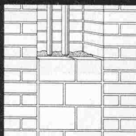
Leitungsschlitz- Isolationen
