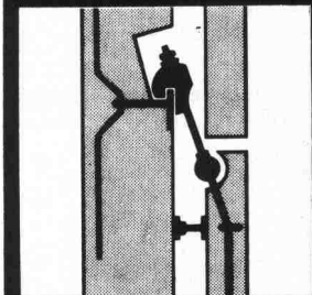
Fassadenplatten-Anker
